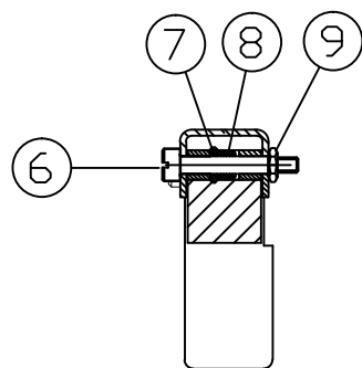
SEZ.A-A
